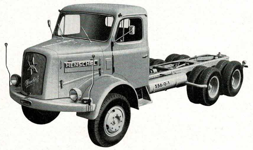
LKW-Fahrgestell 6 x 6
